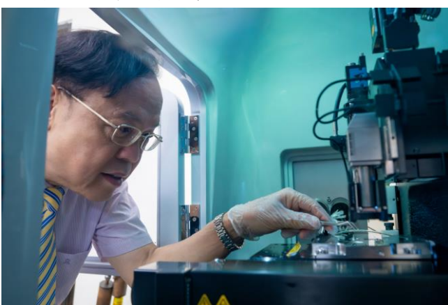
葉均蔚教授將高熵合金放進奈米壓痕機械性質分析儀，測試高熵薄膜硬度。
